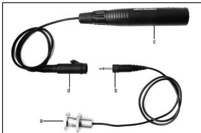
Abb. 1: C 562 CM und Phantomspeseadapter
